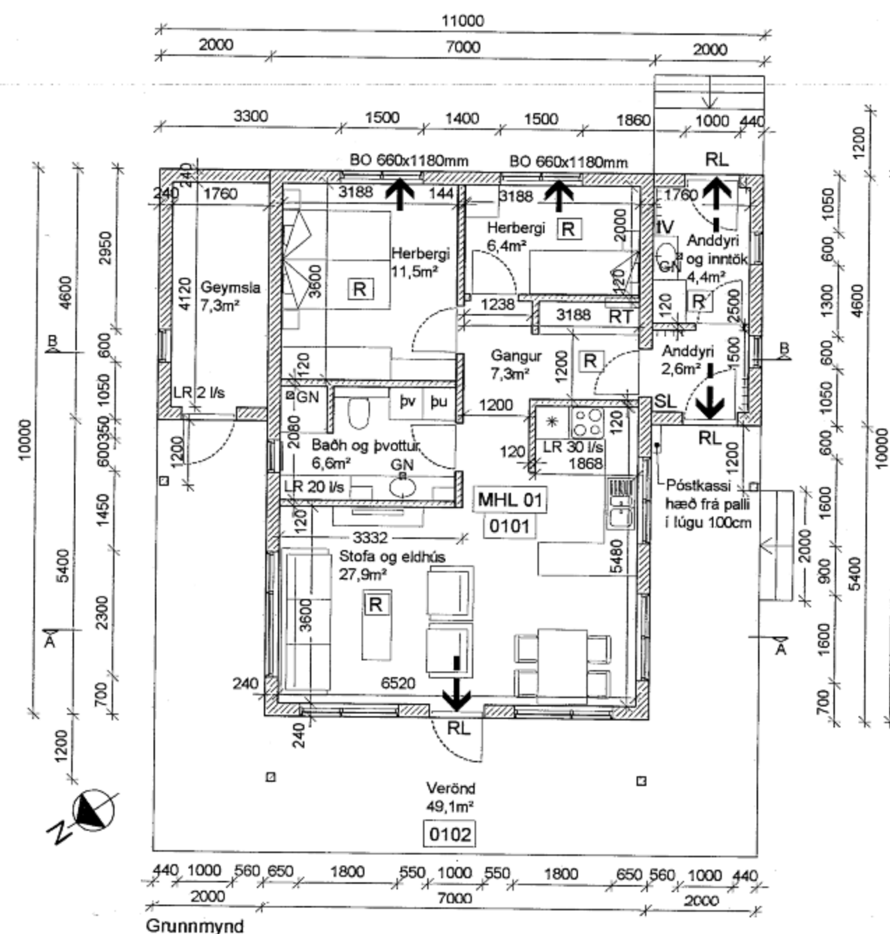
Grunnmynd
