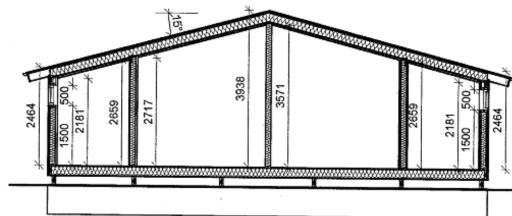
Snið B-B
