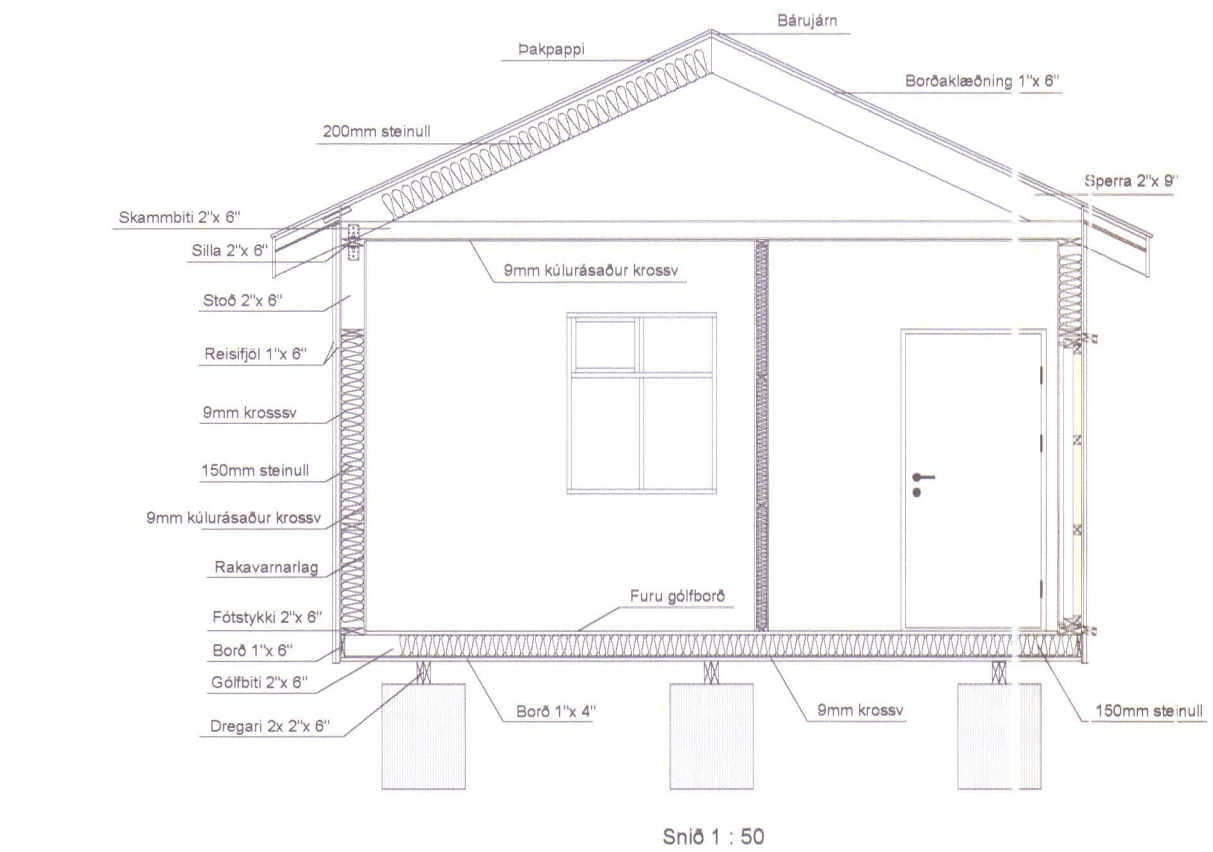
Snið 1 : 50
