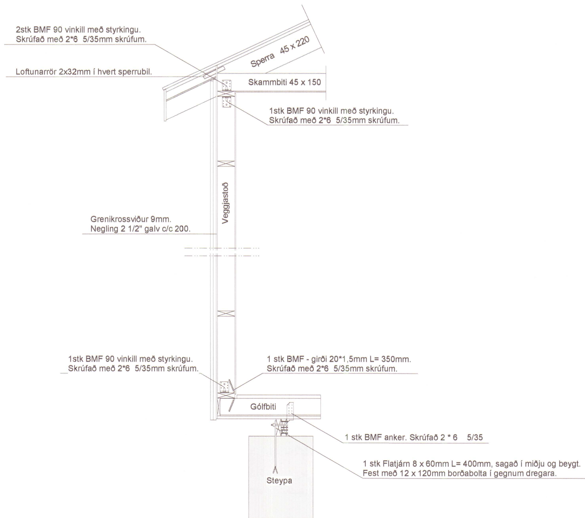
Deili 1 : 20
