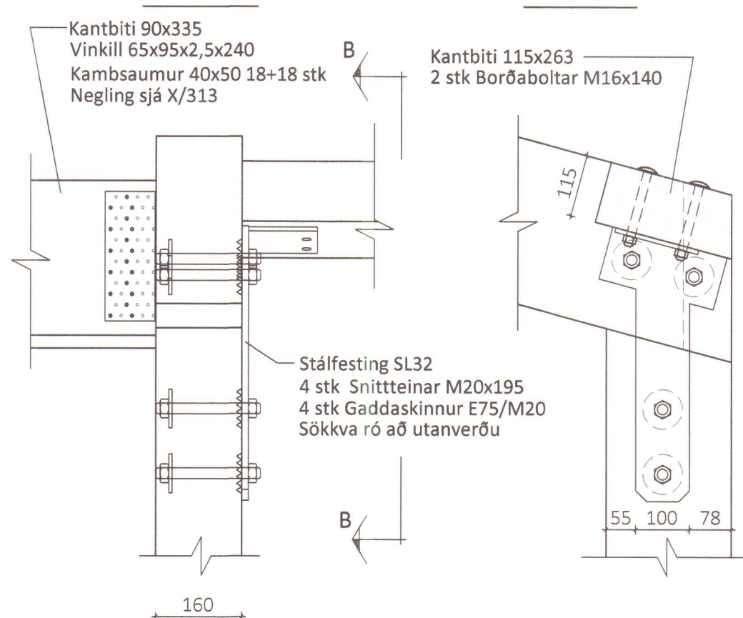
Sniở B-B
