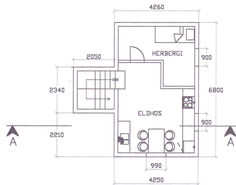
GRUNNMYND KJALLARI
