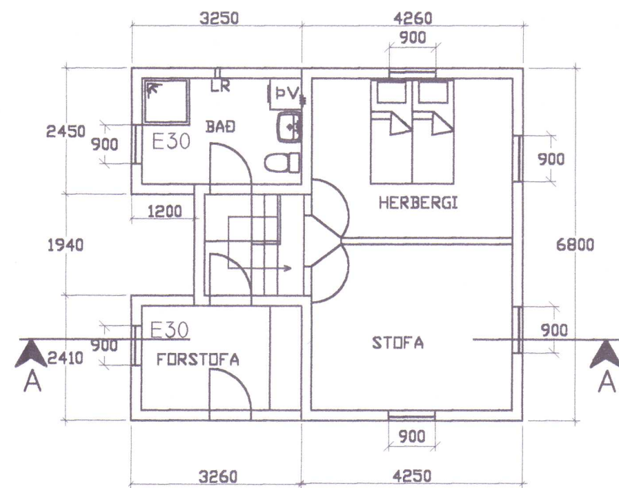
GRUNNMYND I.HÆÐ
