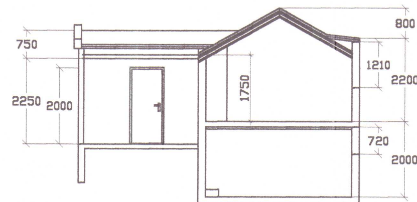
SNIÐ A-A
