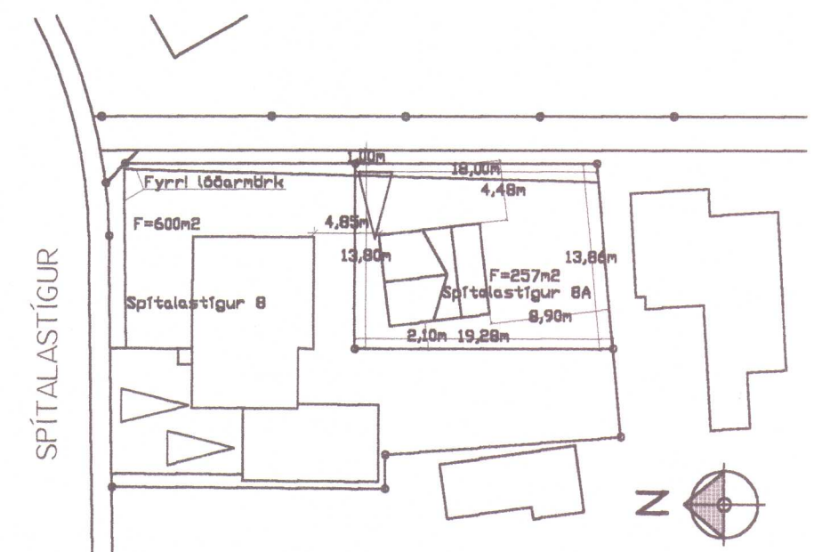
AFSTÖÐUMYND MKV. 1:500
