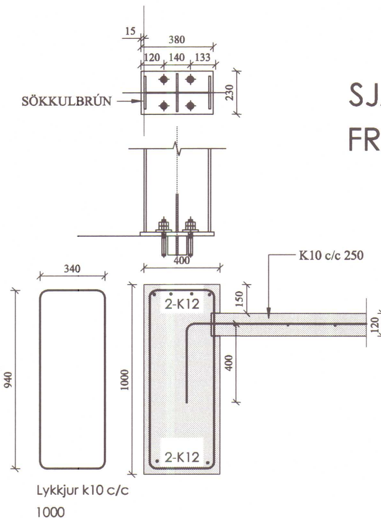
SNID A MK. 1:20
