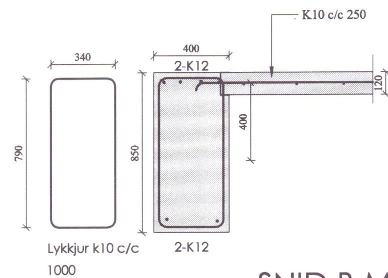
SNID B MK. 1:20
