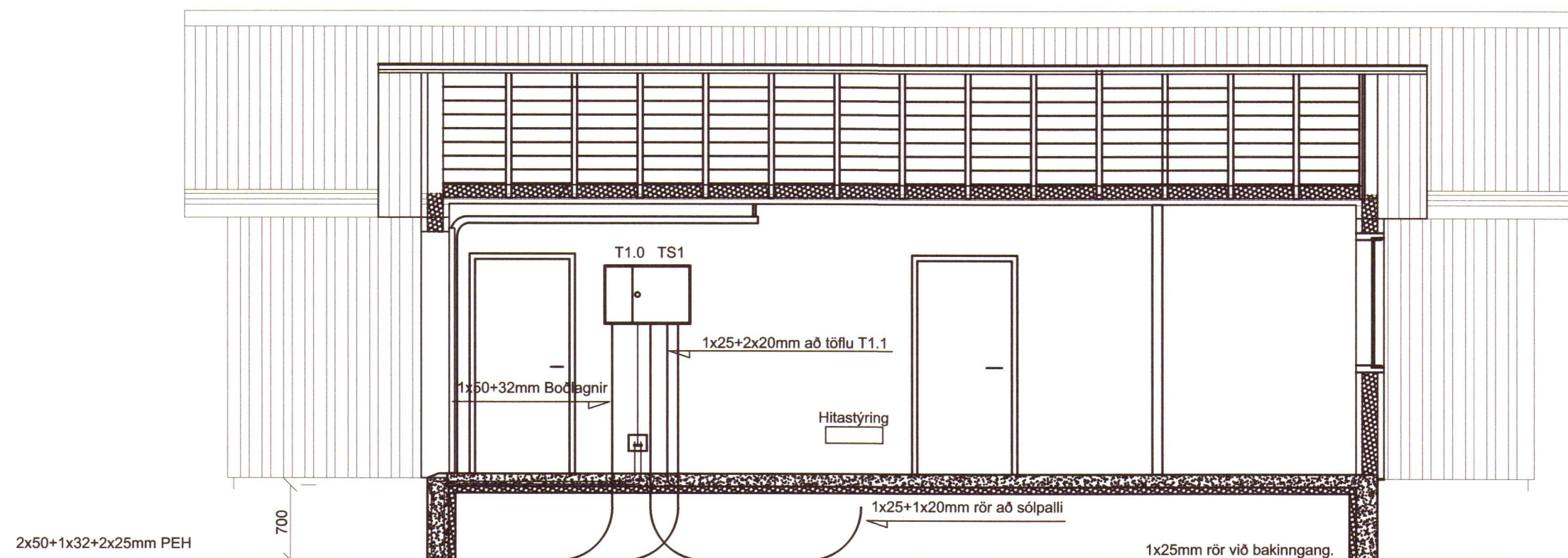
SNID A-A mkv 1:50
