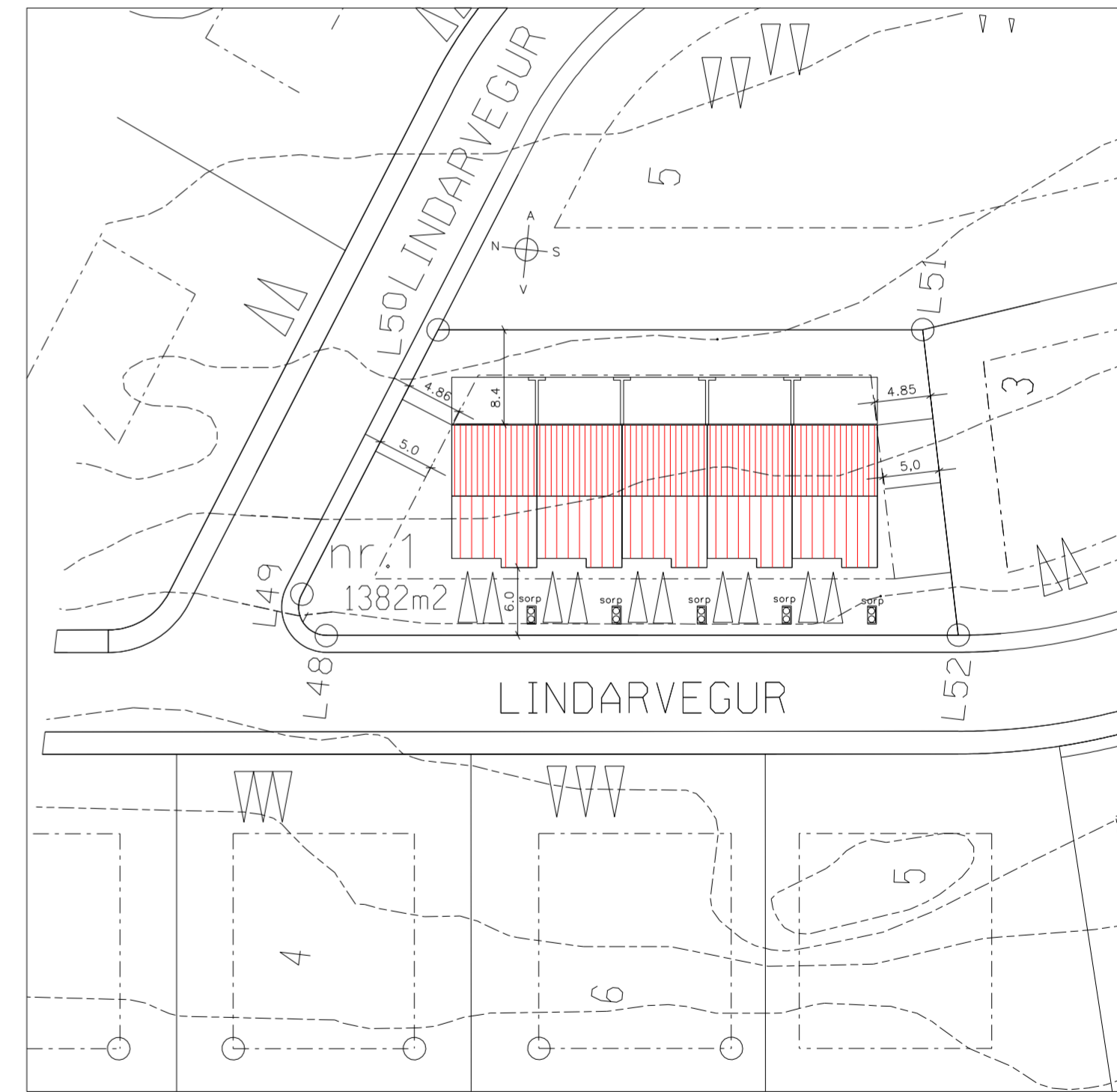
AFSTÖÐUMYND MK. 1:500
